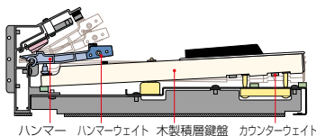
ハンマー ハンマーウェイト 木製積層鍵盤 カウンターウェイト
